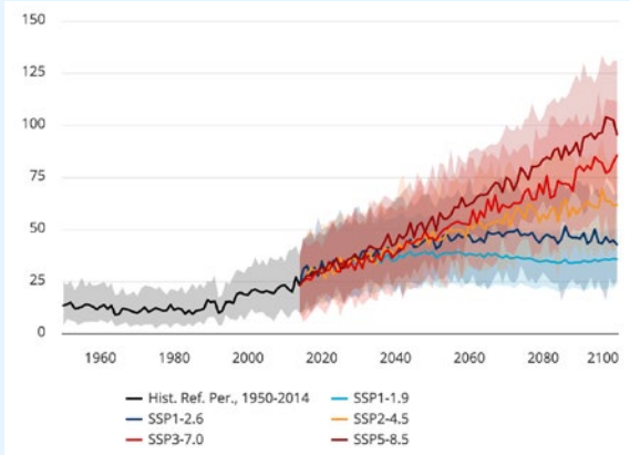
不同情景下——預計熱指數>35℃的天數分佈圖
